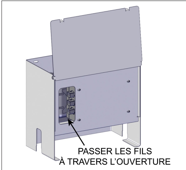
FIGURE 79: BRANCHER LE HARNAIS DES DEUX VÉRINS MOTORISÉS À LA BOITE DE COMMANDE
