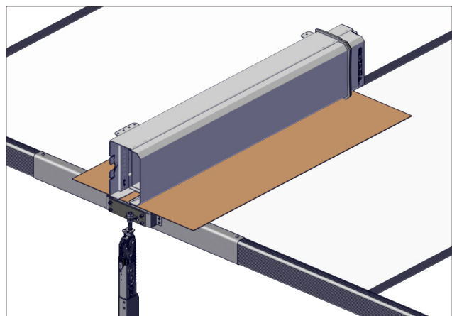
FIGURE 63: PLACER UN MORCEAU DE CARTON (OU PANNEAU DUR DU CAISSON) SUR LE PROFILÉ EN I ET Y DÉPOSER UN DES ASSEMBLAGES DE MANCHONS
