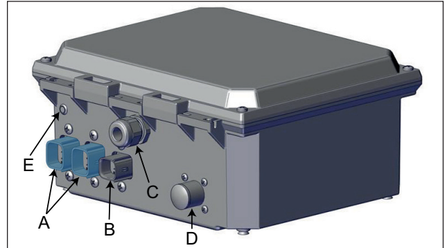
FIGURE 75: BRANCHER LE HARNAIS DES DEUX VÉRINS MOTORISÉS À LA BOITE DE COMMANDE À C.A. (VOIR LA SECTION DES DIAGRAMMES ÉLECTRIQUES)
