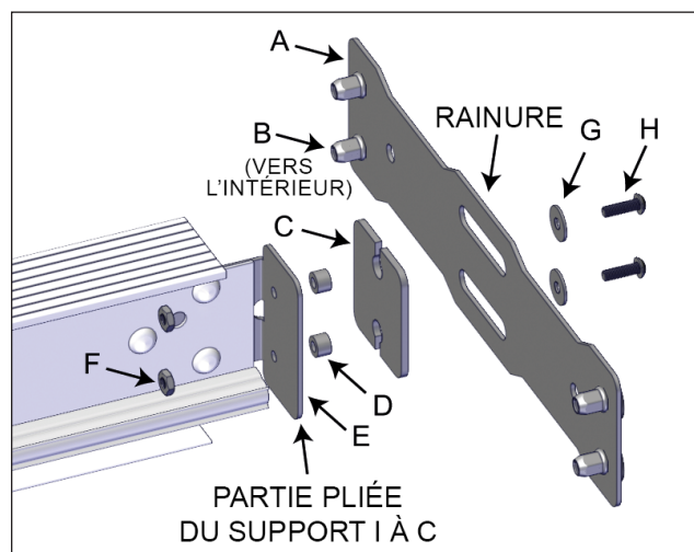
FIGURE 6: INSTALLER LES PLAQUES DE FIXATION LONGUES I À C
