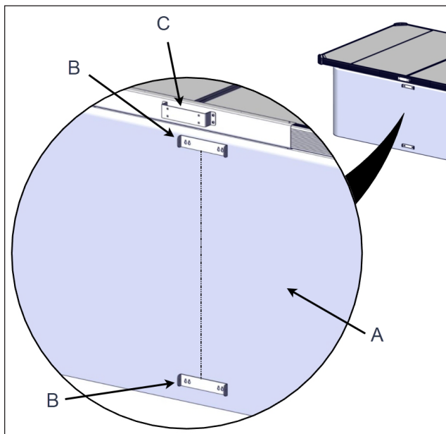
FIGURE 51: POSITIONNER LES SUPPORTS DE MONTAGE SELON LES REPÈRES DE RUBAN-CACHE ET LES FIXER AVEC LES VIS APPROPRIÉES
