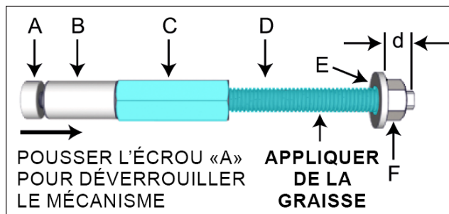
FIGURE 33: INSÉRER LE GOUJON CREUX DANS L'ÉCROU D'ACCOUPLLEMENT HEXAGONAL JUSQU'À CE QU'IL ATTEIGNE L'EXTRÉMITÉ DU GRIPLOCK
