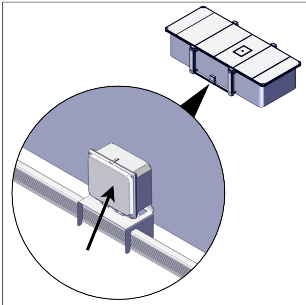
FIGURE 74: PLACER LA BOITE DE COMMANDE ET SON SUPPORT SUR UN DES PROFILÉS EN U, ENTRE LES MANCHONS
