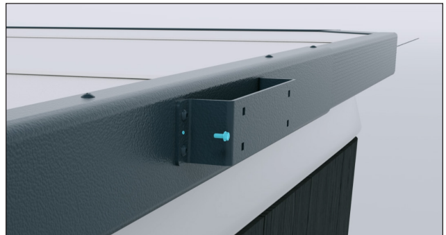
FIGURE 44: VISSER UNE VIS TRANCHANTE DE 3/8 PO DU CÔTÉ INTERNE DE CHAQUE SUPPORT DE MONTAGE
