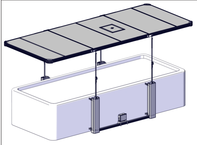
FIGURE 126: VAPORISER LA GRAISSE SUR TOUTES LES PARTIES COULISSANTES ET SUR LES COMPOSANTS MÉCANIQUES DE CHAQUE VÉRIN
