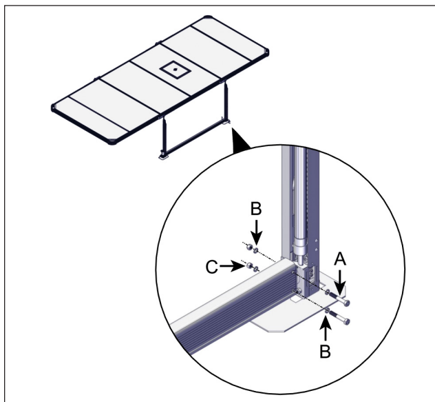
FIGURE 57: INSTALLER LE PROFILÉ EN U AU-DESSUS DE L'ARBRE D'ENTRAÎNEMENT TUBULAIRE ET LE FIXER EN PLACE
