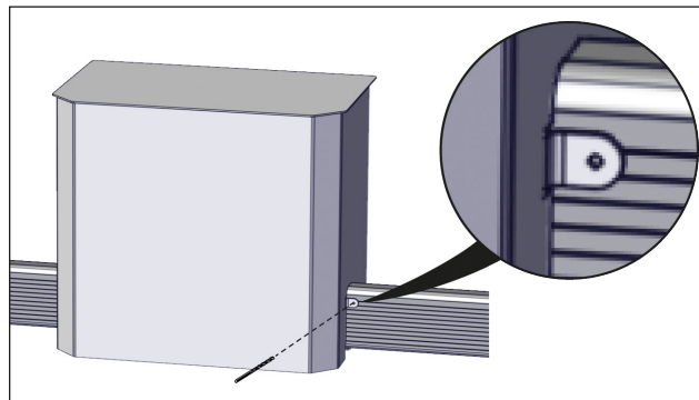
FIGURE 84: PERCER UN TROU À TRAVERS LA LANGUETTE ET DANS LE PROFILÉ EN U (AVEC LE FORET 5/32 PO). VISSER UNE VIS TRANCHANTE À TÊTE HEXAGONALE 8-32 X 3/8 PO
