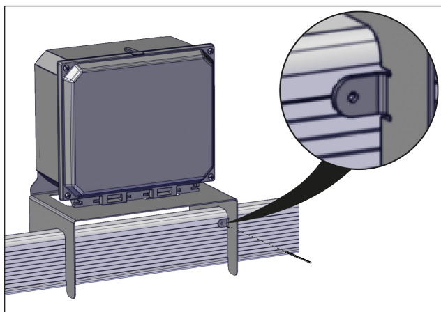
FIGURE 77: PERCER UN TROU À TRAVERS LA LANGUETTE SUR LE SUPPORT DE LA BOÎTE ET DANS LE PROFILÉ EN U (AVEC LE FORET 5/32 PO). VISSER UNE VIS TRANCHANTE À TÊTE HEXAGONALE 8-32 X 3/8 PO
