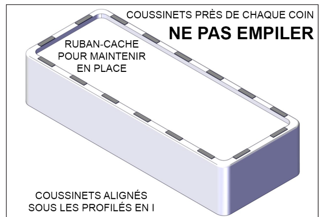
FIGURE 4: INSTALLER LES COUSSINETS PROTECTEURS
