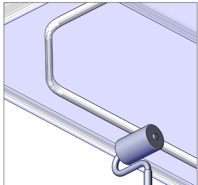
FIGURE 110: APPLIQUER UNE PRESSION DE 7 KG/CM² SUR LE JOINT AVEC LE ROULEAU
