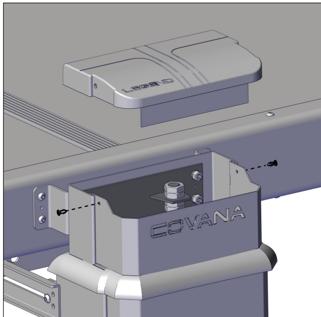
FIGURE 122: RETIRER LES DEUX RIVETS POUSSOIRS DE LA PLAQUE SUPÉRIEURE DE CHAQUE COLONNE
