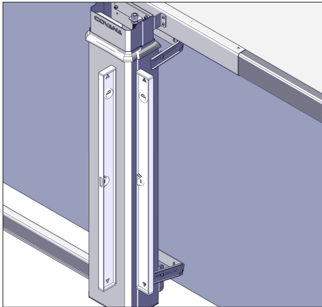
FIGURE 68: UTILISER UN NIVEAU DE 92 CM (36 PO) DE LONGUEUR POUR S'ASSURER QUE LES 4 COLONNES SONT PARFAITEMENT VERTICALES
