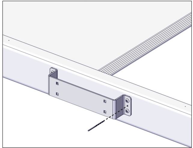
FIGURE 43: CÔTÉ INTERNE DE CHAQUE SUPPORT DE MONTAGE
