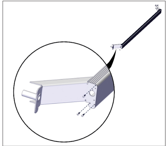
FIGURE 29: INSTALLER UN SUPPORT DE COIN DROIT ET UN GAUCHE SUR CHAQUE PROFILÉ EN C DE BOUT AVEC TROIS VIS AUTOTARAUEUSES N° 8 X 1/2 PO
