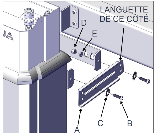
FIGURE 69: FIXER LES BRAS SUPÉRIEURS DU SUPPORT DE MONTAGE AU SUPPORT DE MONTAGE DU SPA
