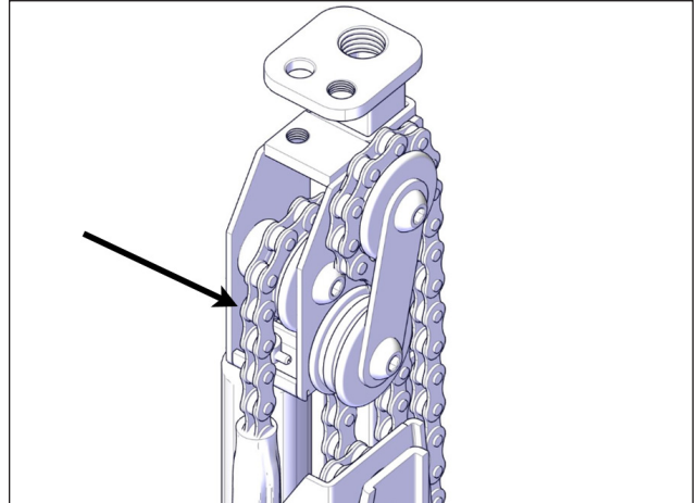
FIGURE 127: INSPECTER LES CHÂÎNES POUR DES SIGNES DE DÉTÉRIORATION
