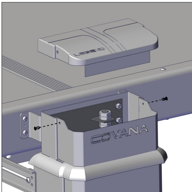
FIGURE 72: INSTALLER UNE PLAQUE SUPÉRIEURE SUR CHAQUE COLONNE À L'AIDE DES 2 RIVETS POUSSOIRS
