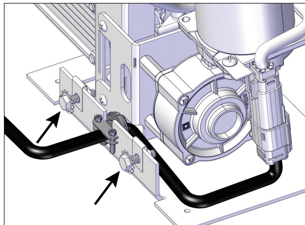
FIGURE 66: GLISSER LES MANCHONS PAR-DESSUS LE VÉRIN ET LES FIXER
