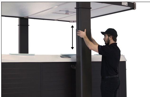
FIGURE 91: ABAISSER LE COUVERCLE ET VÉRIFIER SI LES MANCHONS SONT DE NIVEAU AVEC UN NIVEAU DE 92 CM (36 PO) SUR LE CÔTÉ ET L'AVANT DES MANCHONS
