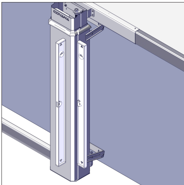
FIGURE 71: VÉRIFIER SI LES COLONNES SONT ENCORE DE NIVEAU DANS LES 2 AXES. SINON, DESSERRER LES BRAS DE MONTAGE ET REPOSITIONNER LES MANCHONS
