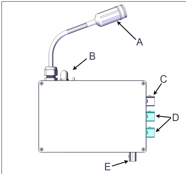
FIGURE 79: BRANCHER LE HARNAIS DES DEUX VÉRINS MOTORISÉS À LA BOITE DE COMMANDE
