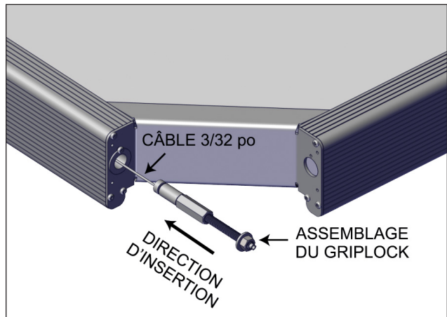
FIGURE 34: ENFILER LE CÂBLE AU TRAVERS DU GRIPLOCK
