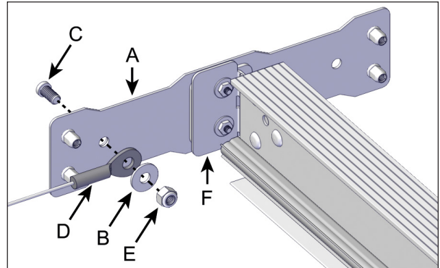
FIGURE 8: INSTALLER LE CÔTÉ PLAT DE L'ŒILLET DU CÂBLE EN CONTACT AVEC LA PLAQUE DE FIXATION LONGUE
