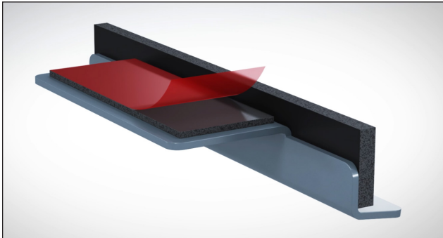
FIGURE 95: RETIRER LE PROTECTEUR ROUGE DE LA BANDE ADHÉSIVE DOUBLE-FACE D'UN JOINT RACLEUR
