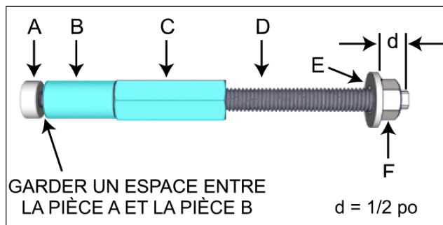
FIGURE 33: INSÉRER LE GOUJON CREUX DANS L'ÉCROU D'ACCOUPLLEMENT HEXAGONAL JUSQU'À CE QU'IL ATTEIGNE L'EXTRÉMITÉ DU GRIPLOCK
