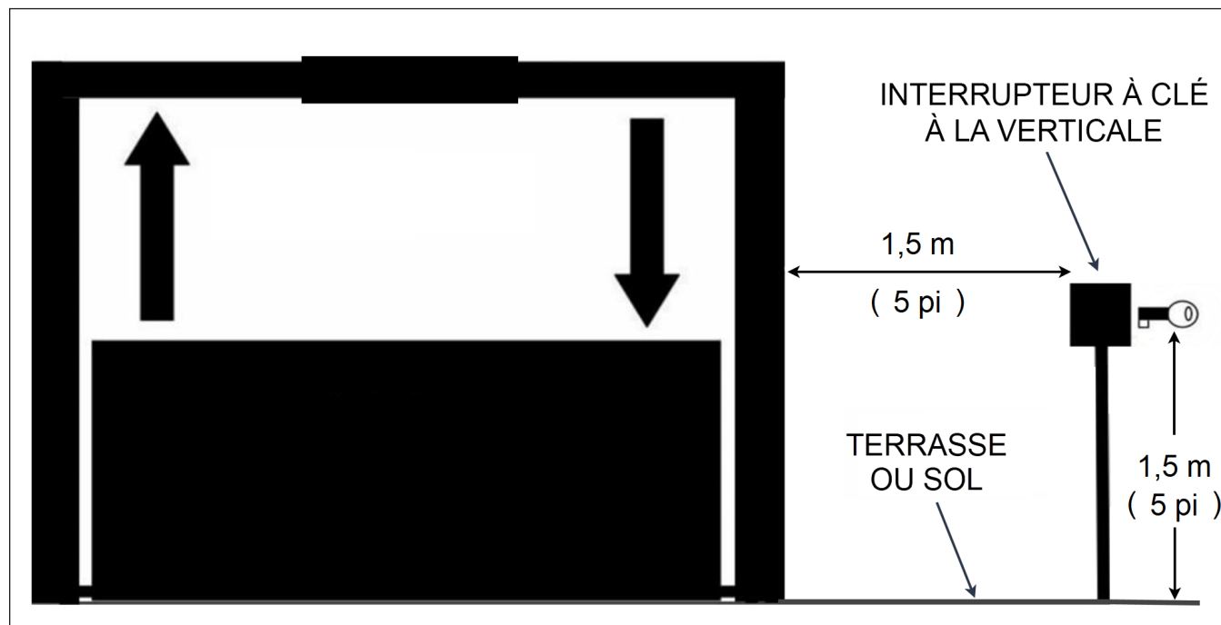
FIGURE 1: EMPLACEMENT DE L'INTERRUPTEUR À CLÉ
