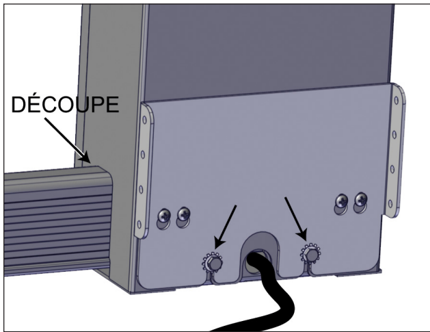
FIGURE 67: SERRER LES DEUX VIS À TÊTE HEXAGONALE À LA BASE DE LA COLONNE (LA RONDELLE PLATE À DOUBLE DENTURE DOIT ÊTRE À L'EXTÉRIEUR DU MANCHON EXTERNE)
