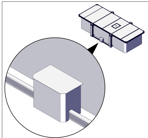
FIGURE 84: PERCER UN TROU À TRAVERS LA LANGUETTE ET DANS LE PROFILÉ EN U (AVEC LE FORET 5/32 PO). VISSER UNE VIS TRANCHANTE À TÊTE HEXAGONALE 8-32 X 3/8 PO
