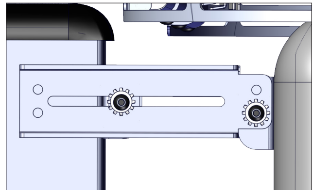
FIGURE 70: VUE LATÉRALE DU BRAS DU SUPPORT DE MONTAGE
