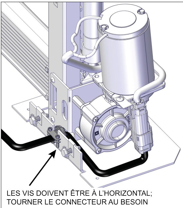
FIGURE 61: SERRER LA BAGUE ET LES VIS DU CONNECTEUR À SELLE
