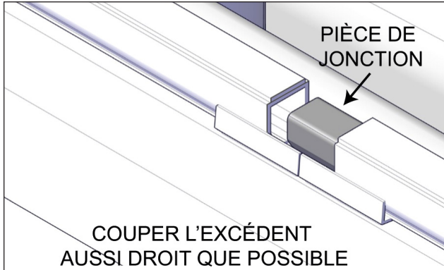
FIGURE 104: INSÉRER LA PIÈCE DE JONCTION DANS LES DEUX EXTRÉMITÉS DU JOINT
