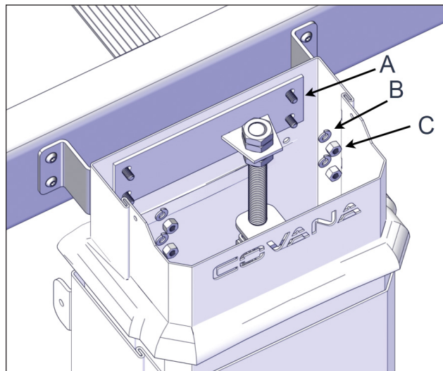
FIGURE 66: GLISSER LES MANCHONS PAR-DESSUS LE VÉRIN ET LES FIXER
