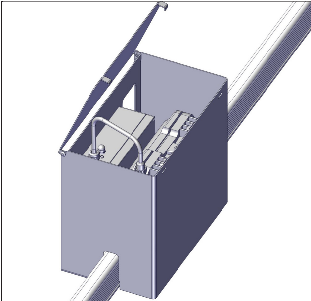
FIGURE 85: OUVRIR LE COUVERCLE DU BOITIER DE LA BOITE DE COMMANDE ET BRANCHER LE HARNAIS DE LA BATTERIE. PLACER LA BATTERIE À L'INTÉRIEUR PUIS FERMER LE COUVERCLE
