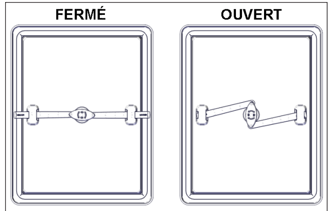
FIGURE 11: RÉTRACTER LES BRAS POUR INSTALLER LA SORTIE D'URGENCE DANS LE PANNEAU CENTRAL
